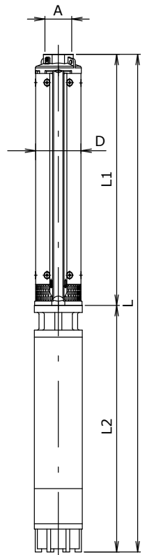
■ 外形図
