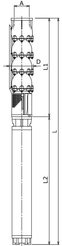
■ 外形図
