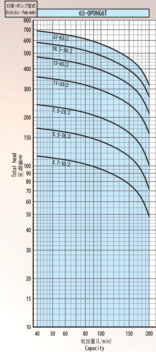
OPDHG6T 50Hz 機種一覧
