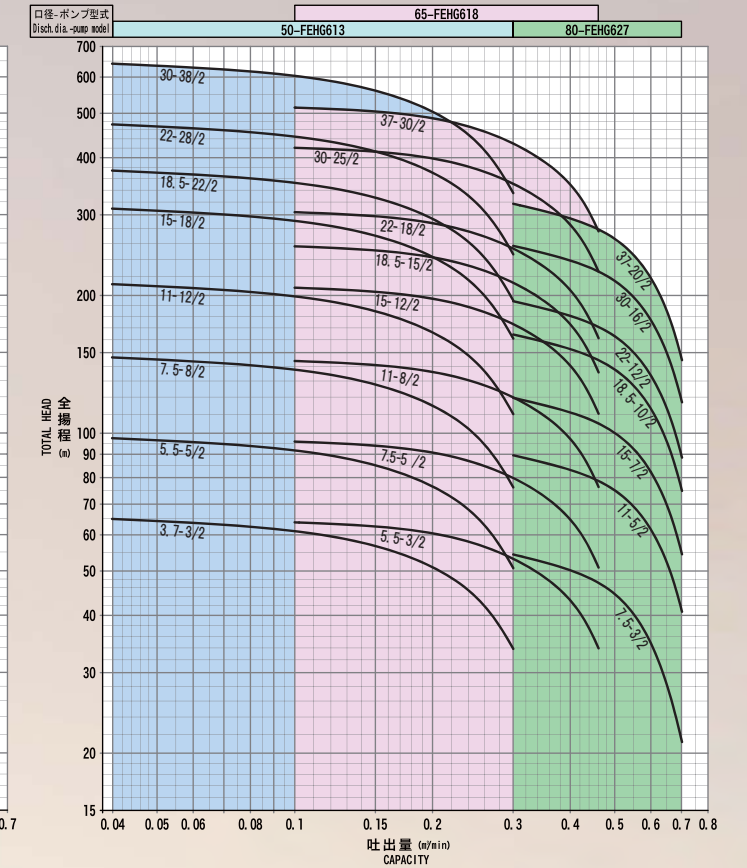
ポンプ選定図FEHG6 60Hz
